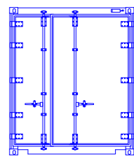
DOOR ELEVATION
